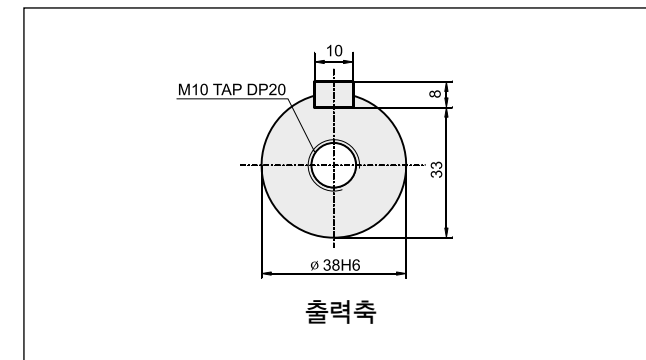
중실축상세도
