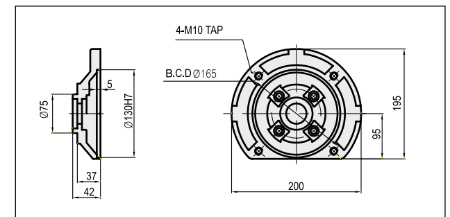
플렌지상세도
