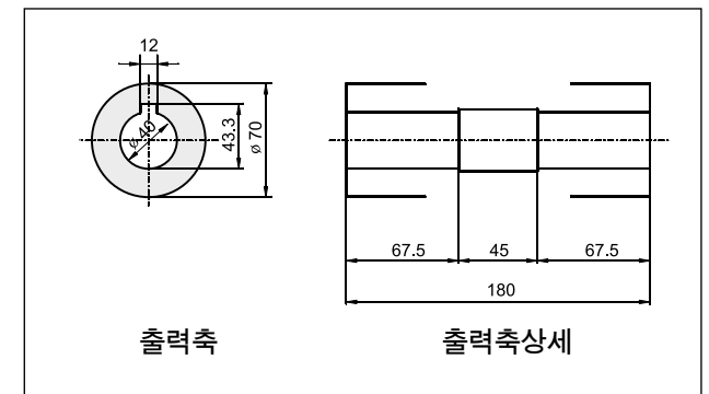
중공축상세도
