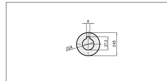
중공입력축상세도
