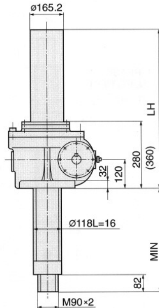
하방향형 Inverted Traveling
