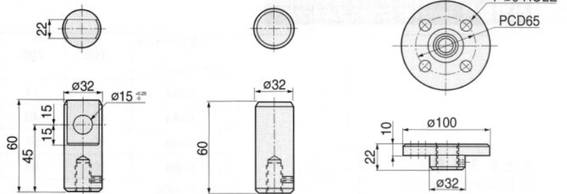
크레비스 너트 Clevis Nut
