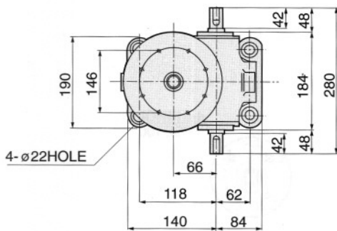
평면도 Plane Figure
