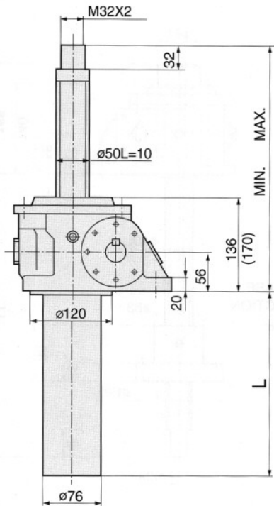
상방향형 Upright Traveling
