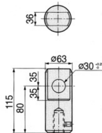
크레비스 너트 Clevis Nut
