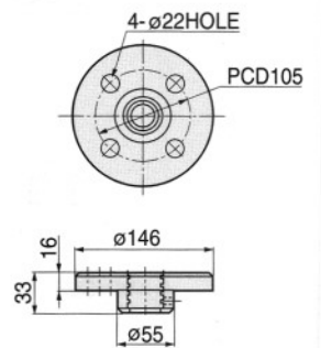
플랜지 너트 Flange Nut
